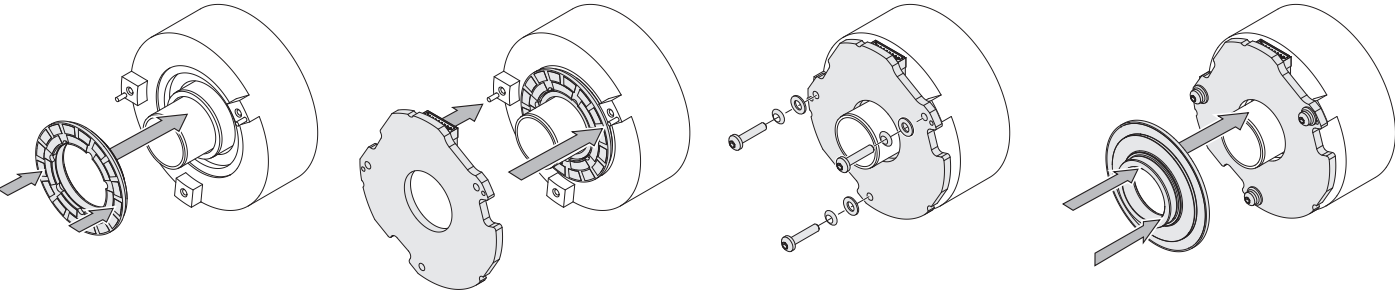
Disco graduato con albero applicato a pressione
