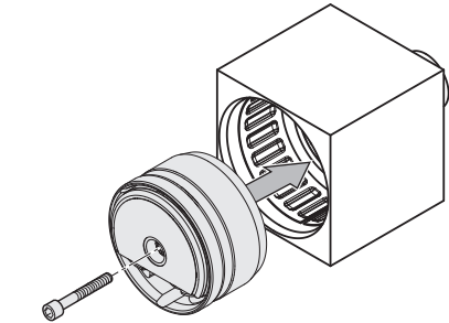
ECI/EQI 1100 con bussola calibrata
