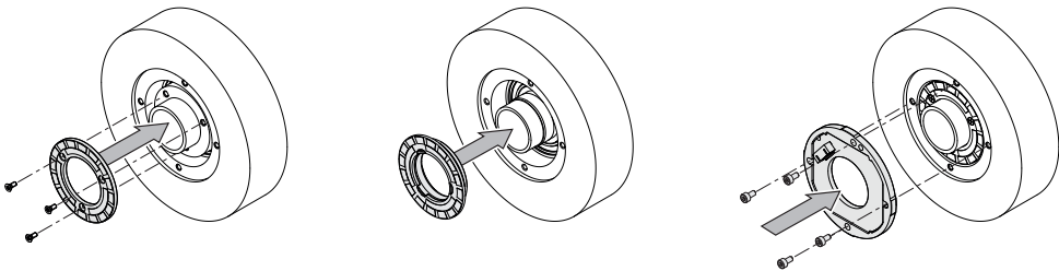
Esempio di montaggio di KCI/KBI 1300
