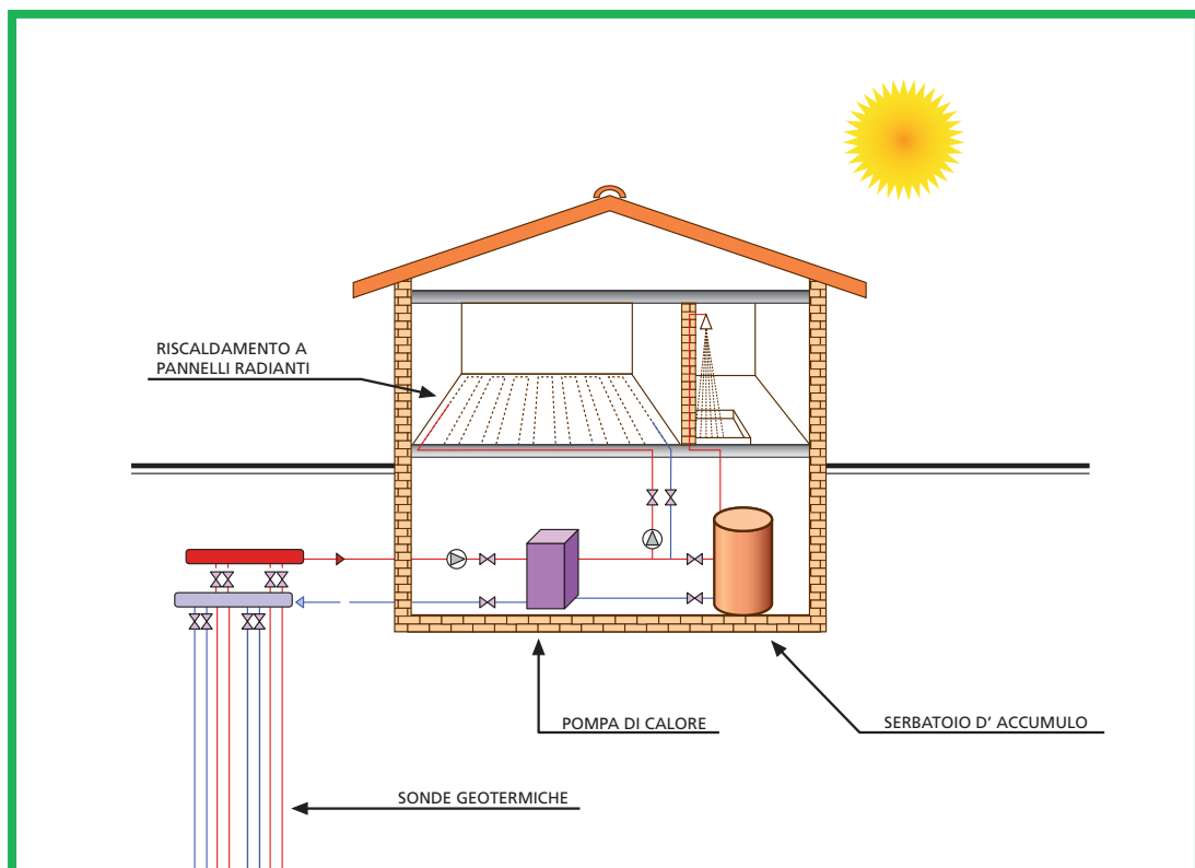
SCHEMA CIRCUITO CHIUSO TERRA/ACQUA (SONDE GEOTERMICHE VERTICALI)
