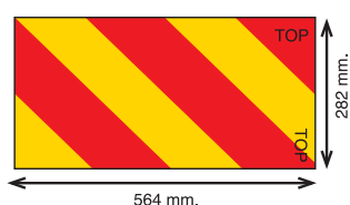
Cod. 90071 Kit 2 pannelli formato 282x564 \nabla 2 mm.
