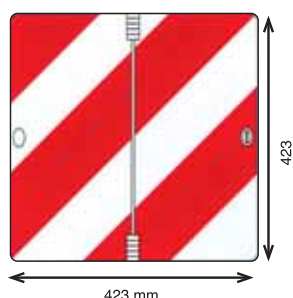
Cod. 90002 Pannello sinistro pieghevole in verticale zincato con angoli arrotondati. 423x423 \nabla 0,8 mm.
