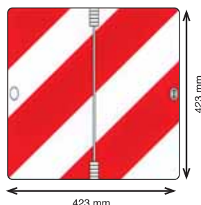
Cod. 90001 Pannello destro pieghevole in verticale zincato con angoli arrotondati. 423x423 \nabla 0,8 mm.
